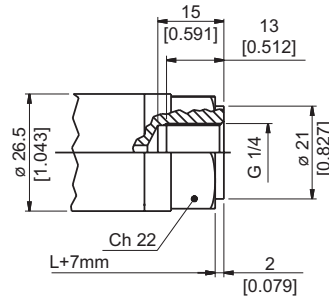
(4) G 1/4 阴纹
