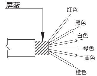
F - 屏蔽电缆 6 x 0.25 - 1m.
