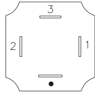
微螺线管 DIN 43650C - ISO4400
